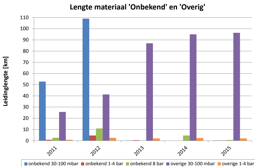
Figuur 4: Ontwikkeling van aandeel onbekende en overig (koper, gerelined gietijzer etc.) leidingmateriaal in de afzonderlijke druknetten.
