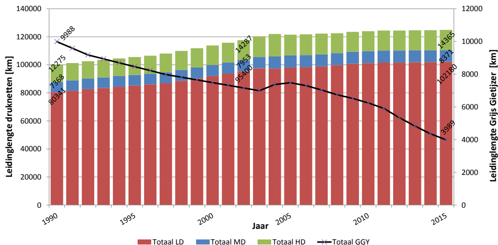
Onderverdeling druknetten en leidinglengte Grijs Gietijzer in Nederland
