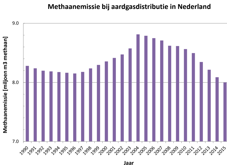
Figuur 1: Trend van de berekende methaanemissie bij aardgasdistributie in Nederland.
